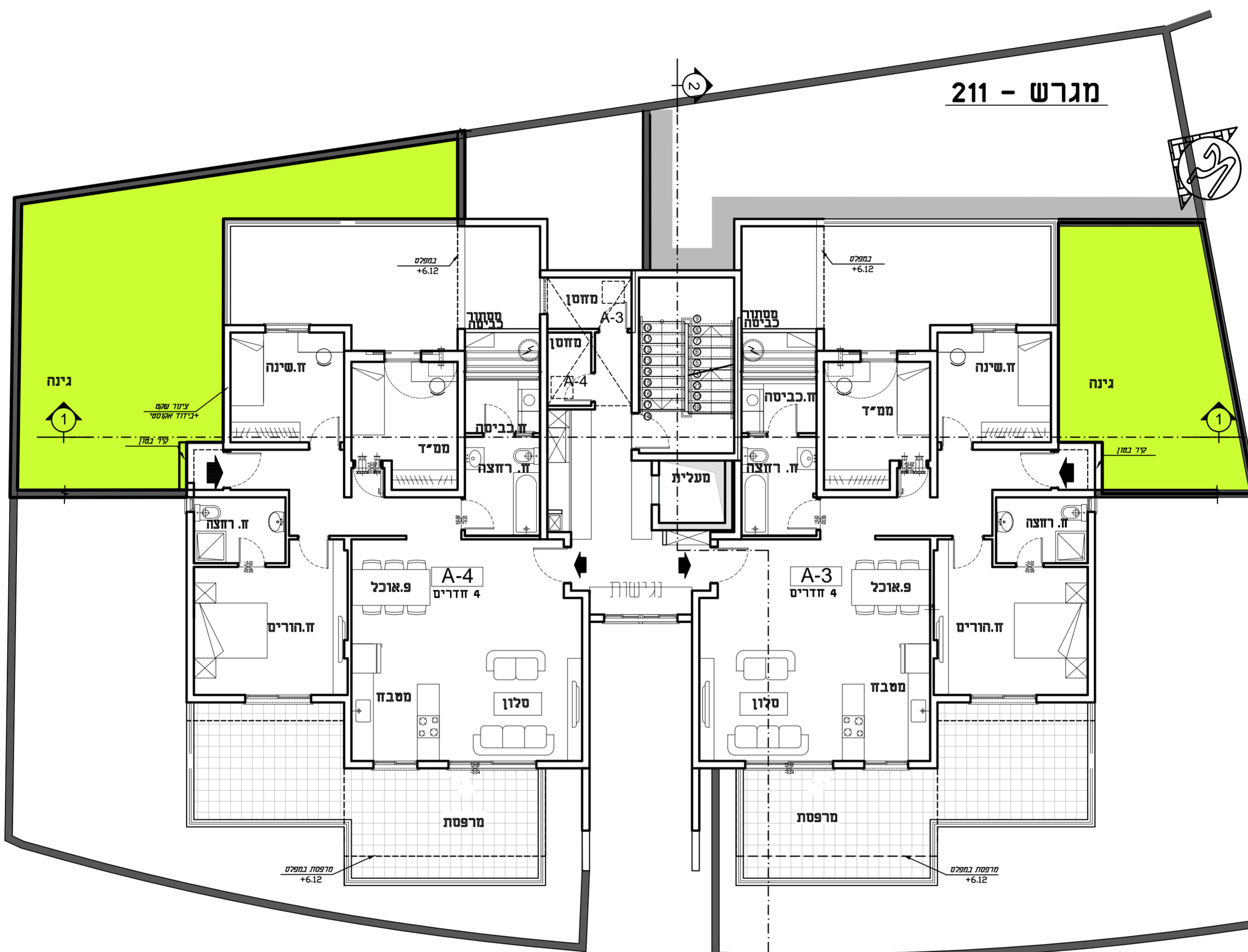
תכנית קומה - א 1:100 מגרש - 211 FL001
