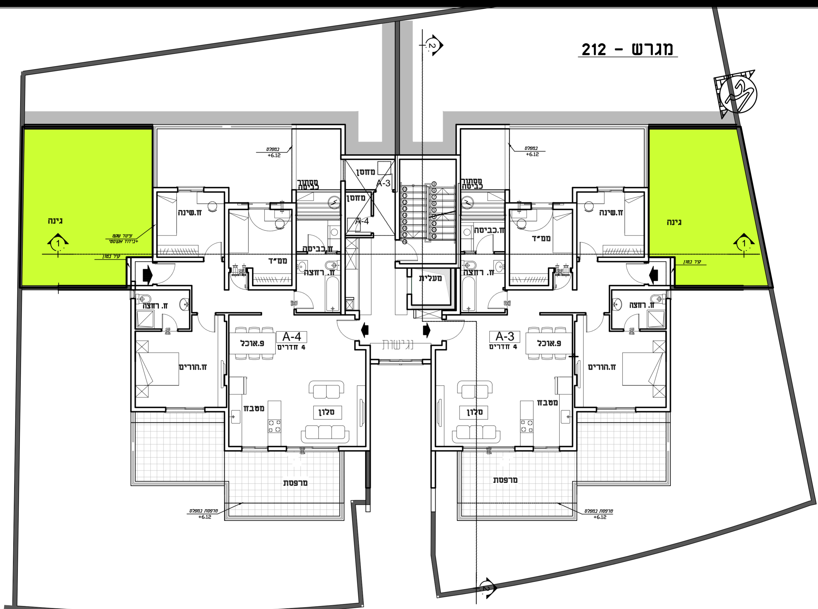
תכנית קומה - א 1:100 מגרש - 212 מפלס : +3.06 FL001
